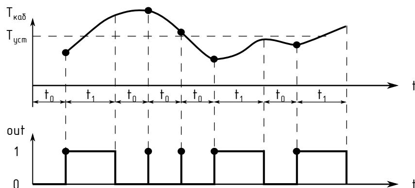
Рисунок 2.5 – Режим работы «По току саморегулирующегося кабеля»
